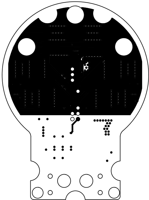
Проводящий рисунок 13
