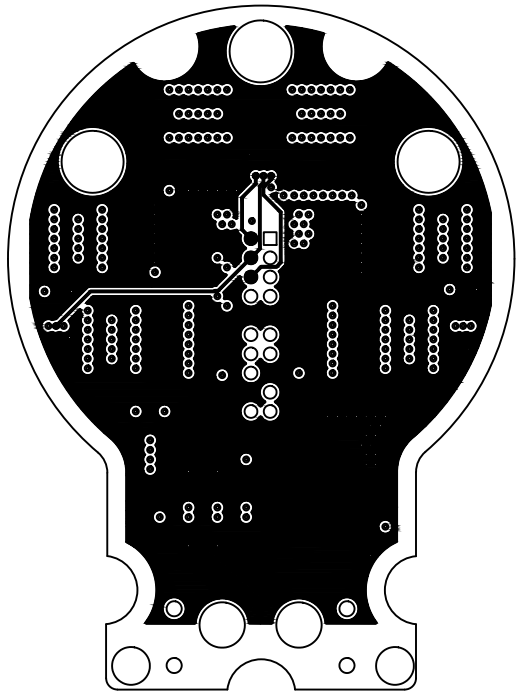
Проводящий рисунок 12
