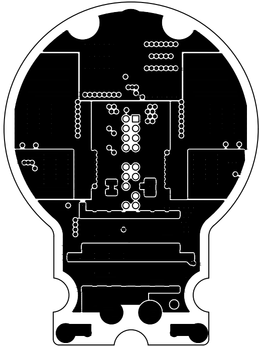
Проводящий рисунок 21
