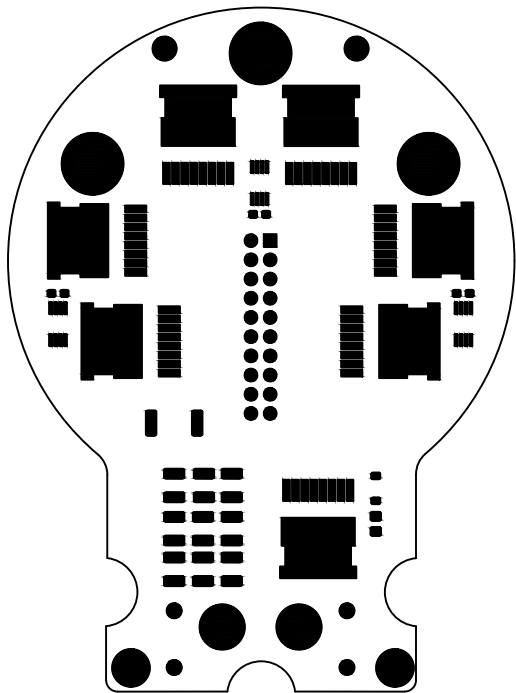
Защитная паяльная маска рисунок 12
