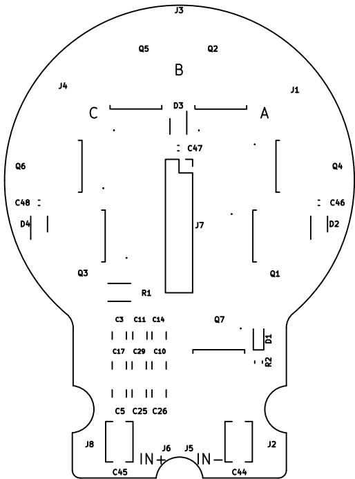
Шелкография рисунок 12
