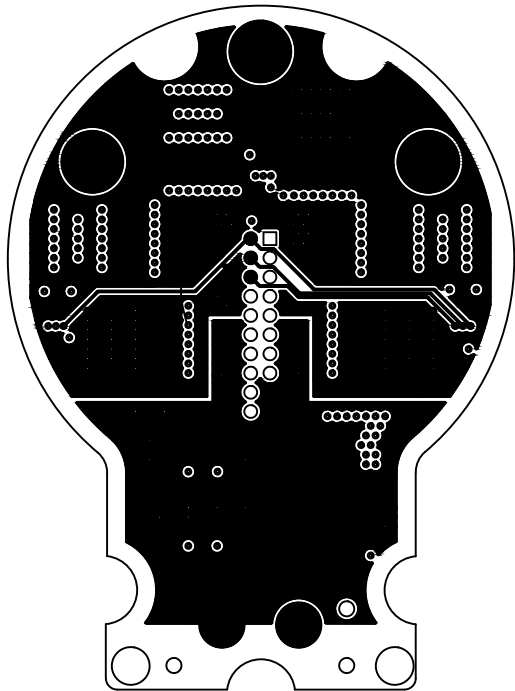
Проводящий рисунок 23
